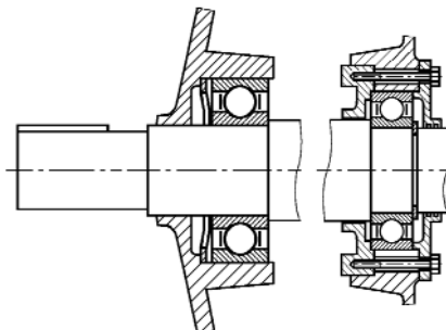
Рисунок 14.2 для двигателей габаритов 160, 180 мм
