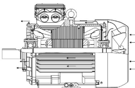
Рисунок 4б Рисунок 4 Двигатели брызгозащищенного исполнения
