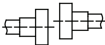
Рис. 2.6.2. Параллельная несоосность
