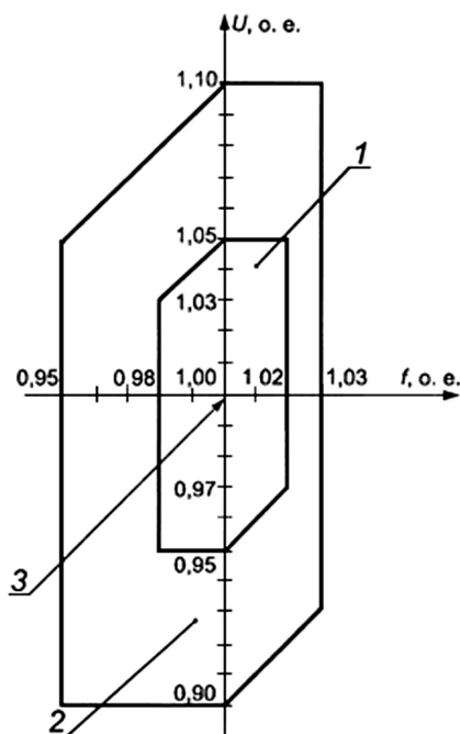
Рис. 2.6.1. Допустимые отклонения параметров сети
