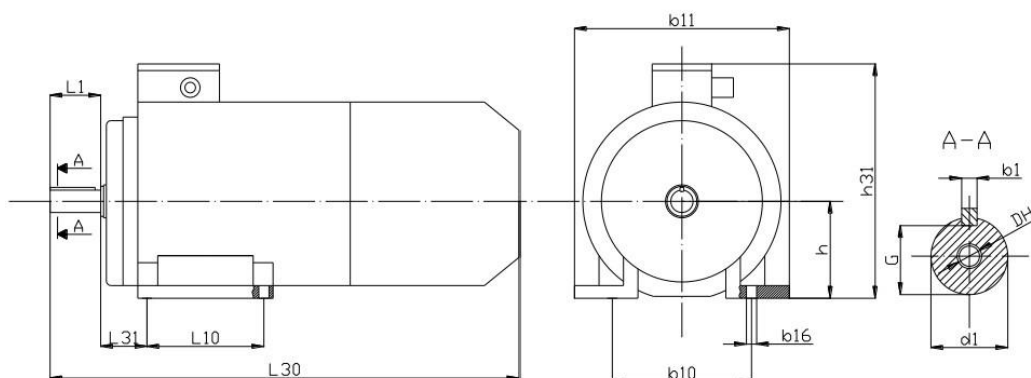
Рис. 9.2. Габаритные и установочно-присоединительные размеры
