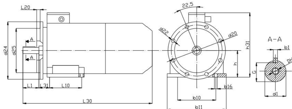
Рис. 9.3. Габаритные и установочно-присоединительные размеры
