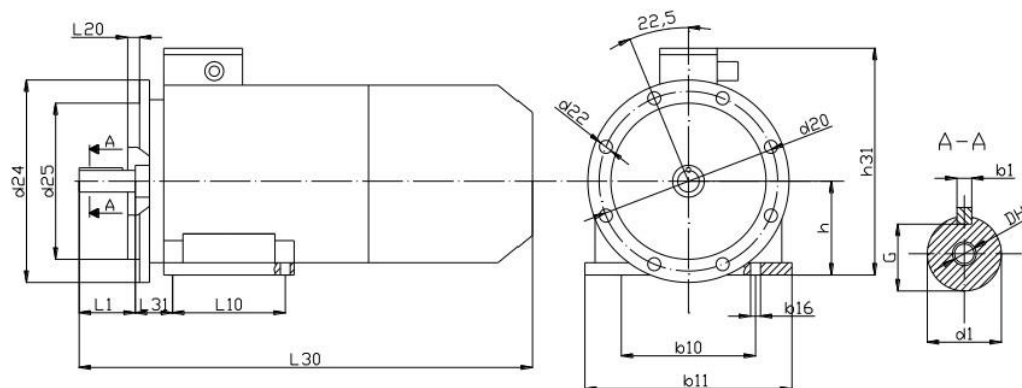
Рис. 9.4. Габаритные и установочно-присоединительные размеры
