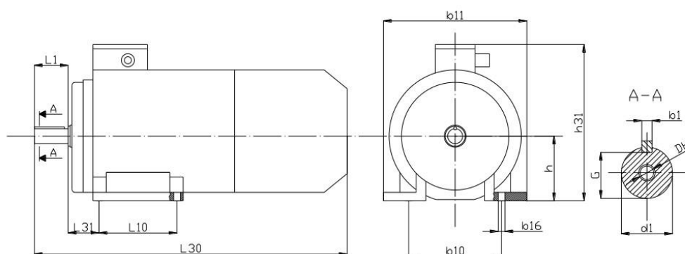
Рис. 9.1. Габаритные и установочно-присоединительные размеры
