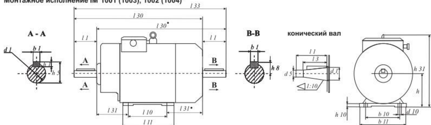
Габаритные, установочные и присоединительные размеры крановых электродвигателей с короткозамкнутым ротором
